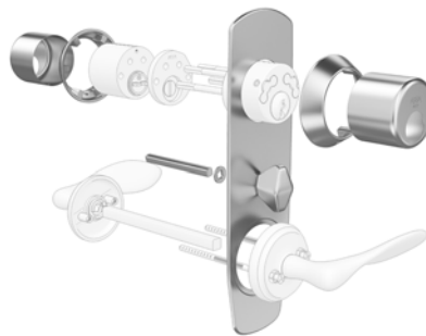
BEHÖRSSATS för rund cylinder och vredskytt
