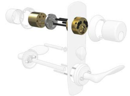
DUBBELCYLINDER 1312 för långskytt, inkl. 5 nycklar
